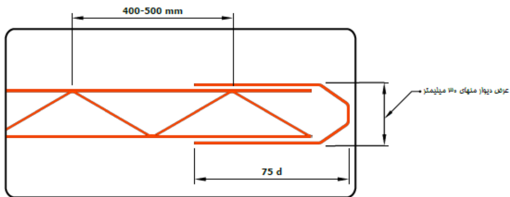
الف- میلگرد بستر خریایی
