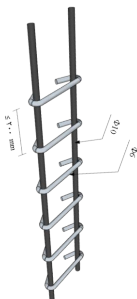
شکل ۸-۱۱- جزئیات شبکه میلگرد کلاف بتنی
