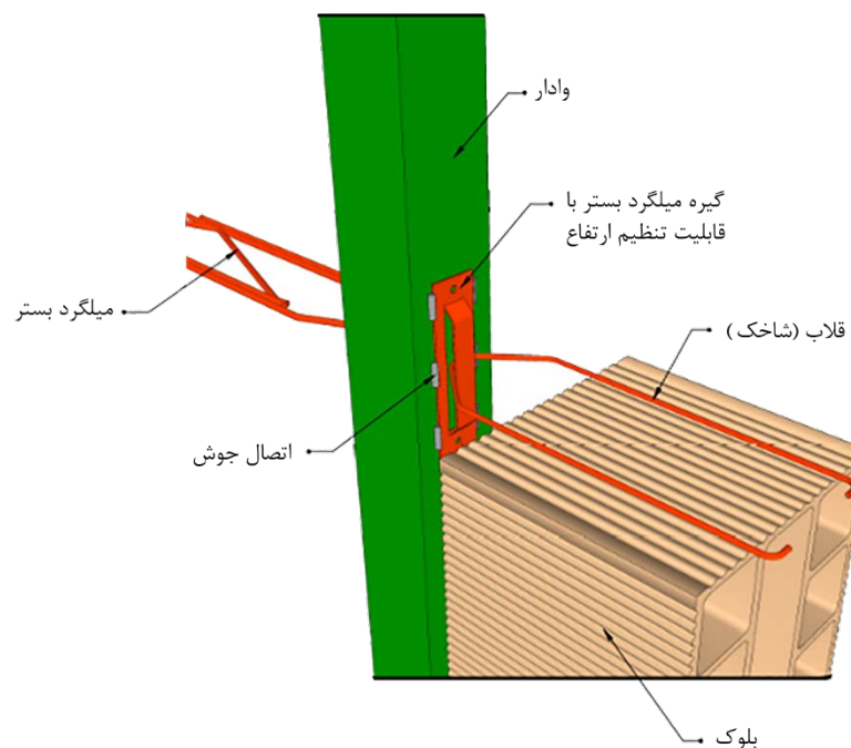
شکل ۸-۳۵- میلگرد بستر در فاصله بین وادارها و اتصال آن به وادار
