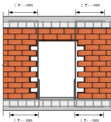
شکل ۸-۹- جزئیات اتصال کلاف بازشوی قائم به کلاف افقی ساختمان
